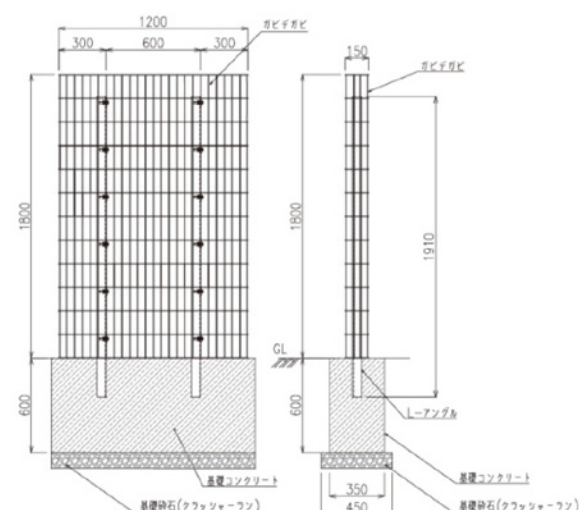
かごウォールH1800単独施工概略図
