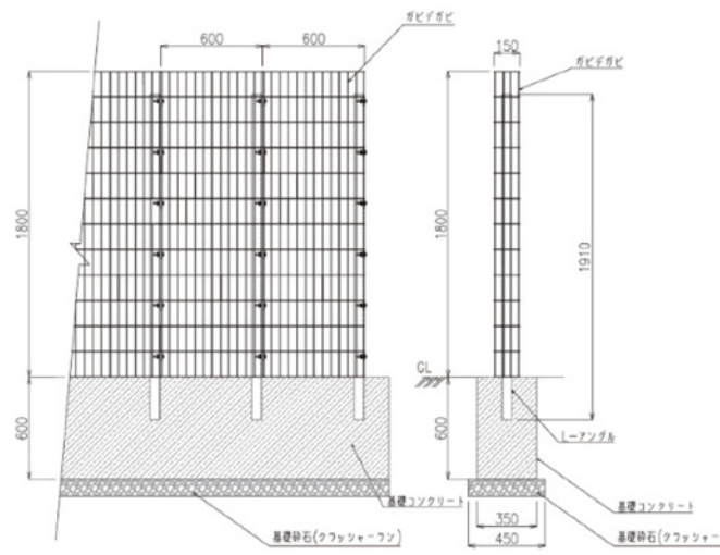
かごウォールH1800連続施工概略図
