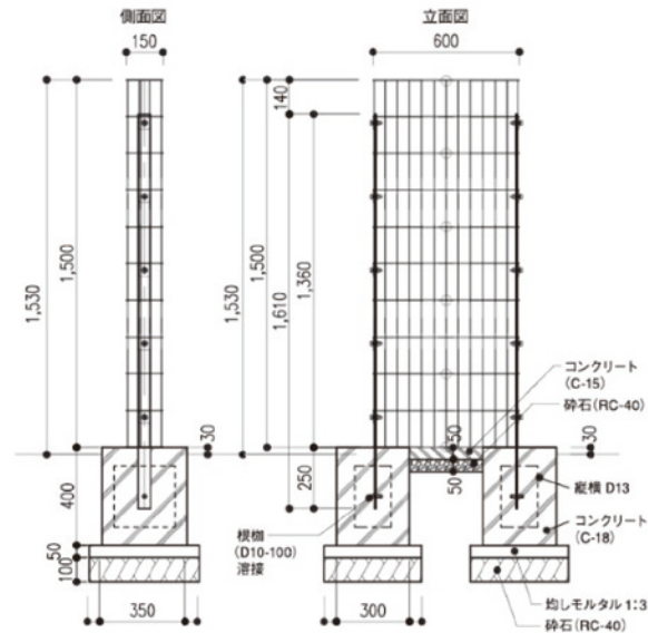
かごウォールH1500推奨基礎図
