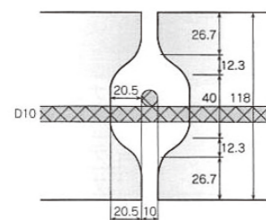
鉄筋を挿入する空洞部寸法
